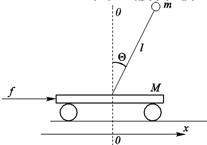
Նկար 3. Մեխանիկական օբյեկտ
